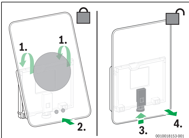
Σχ. 7 Τοποθέτηση/αφαίρεση θερμοστάτη
