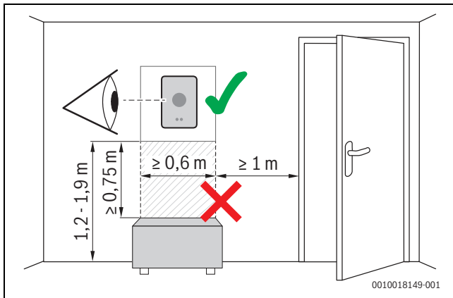
Σχ. 3 Θέση εγκατάστασης θερμοστάτη, απόσταση
